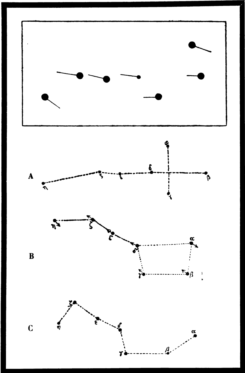
Рис. 5. Собственные движения звезд Большой Медведицы и изменения ее конфигурации. А — какой она была за 50 000 лет до нашего времени, В — теперь, и С — через 50 000 лет.
