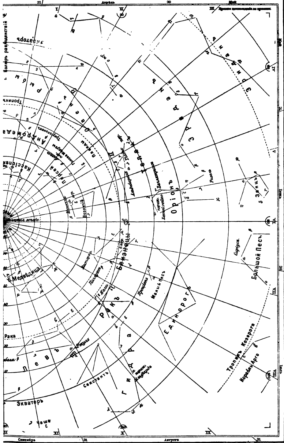
ых затмений, указанных в таблицах II главы. Координаты даны для эпохи 1900 года столбцами «прямо над соответствующими «часам» (и таблицей на стр. 136 в IV книге га»).
