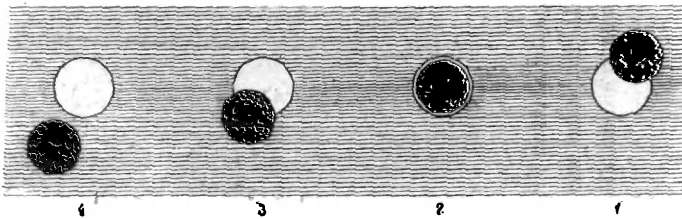
Рис. 20. Ход кольцеобразного затмения Солнца в нисходящем узле лунной орбиты.
