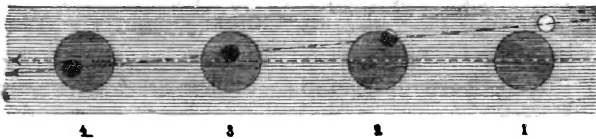
Рис. 9. Лунное затмение у нисходящего узла лунной орбиты.
