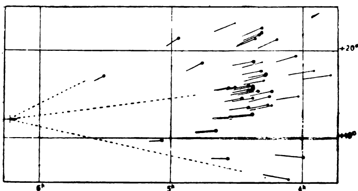
Рис. 6. Собственное движение Гиад среди соседних крупных звезд.
