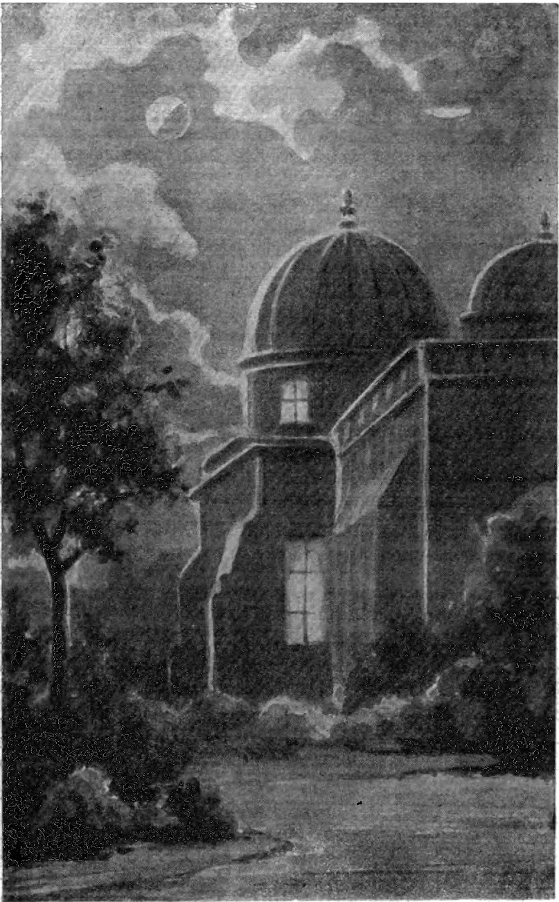
Рис. 10. Начало кровавого лунного затмения, когда вместо полного потемнения происходит, благодаря рефракции солнечных лучей в земной атмосфере, лишь преобразование Луны в красный вид.
