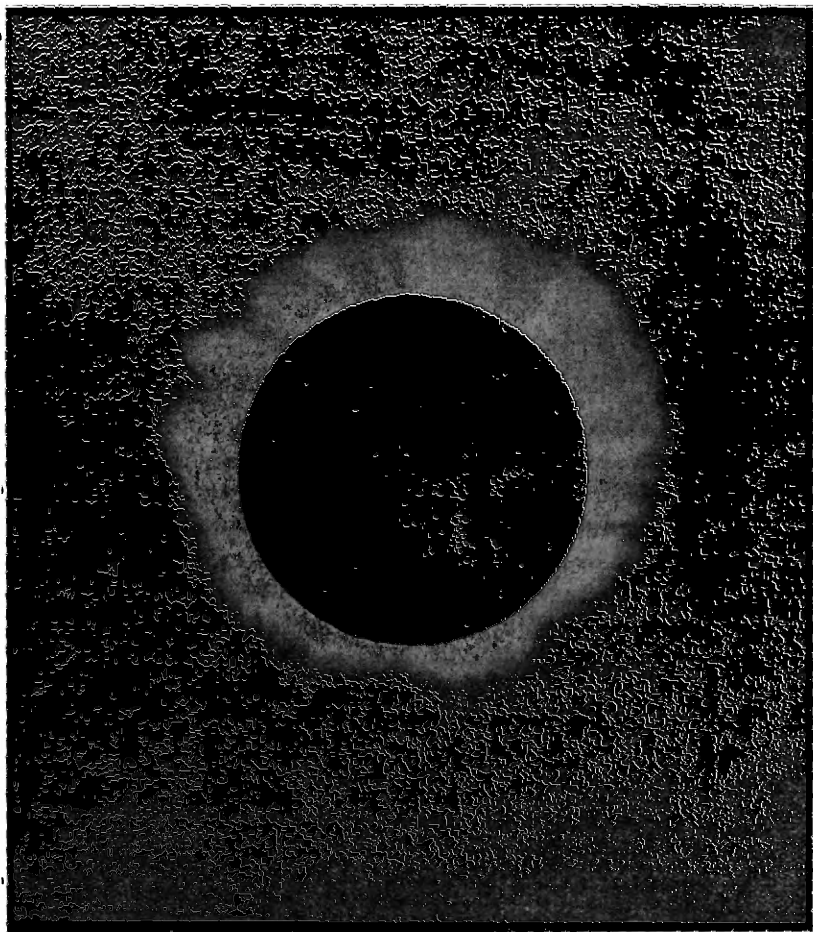
Рис. 16. Вид солнечной короны при полном затмении в период минимума пятнообразовательной деятельности Солнца.
