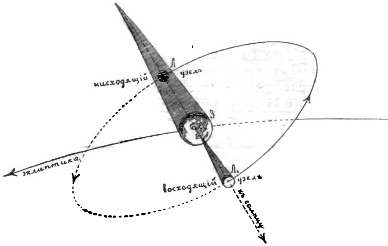
Рис. 7. Центральное лунное и солнечное полные затмения, обычно совершающиеся через 14 дней одно после другого.
