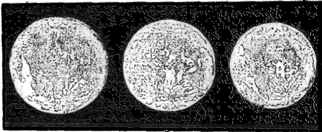
Рис. 11. Сравнительная кажущая величина Луны на ближайшем, на среднем, и на дальнейшем расстоянии от Земли.
