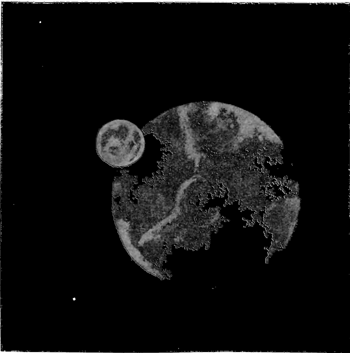
Рис. 23. Каким видно с Солнца начало солнечного затмения на Земле.
