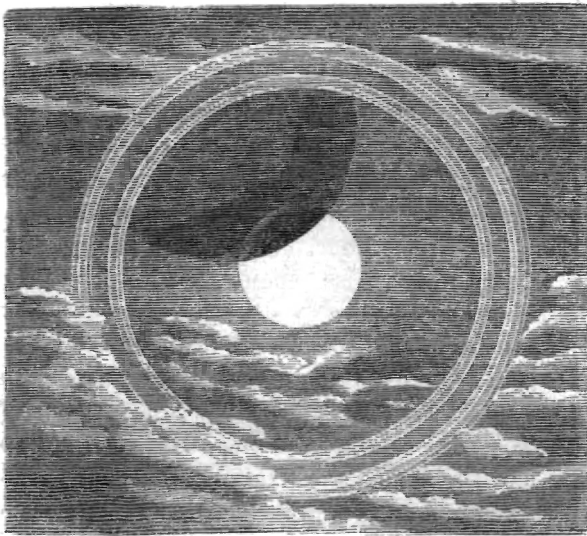
Рис. 44. Лунное затмение, окруженное галосом.
