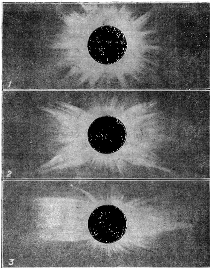
Рис. 22. Три вида солнечной короны во время полных солнечных затмений. 1. — Во время минимума пятнообразовательной деятельности Солнца. 2. — В промежуток между максимумом и минимумом и 3. — Во время максимума пятнообразовательной деятельности.
