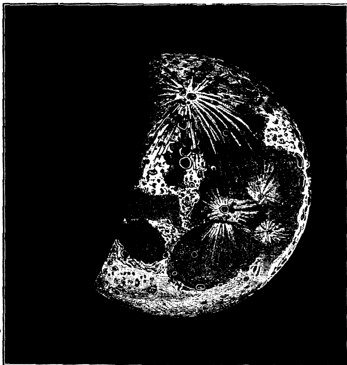
Рис. 12. Перед окончанием полного черного лунного затмения 4 октября 1884 г., когда полутень имела голубой цвет (тогдашний рисунок).
