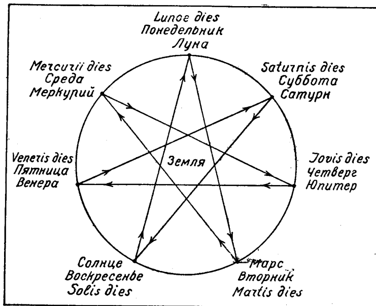
Рис. 149. Скалигерова звезда.
