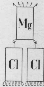
Иллюстрація 85. Хлористый магній.
