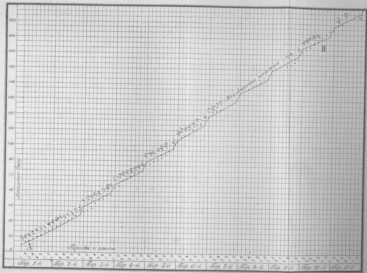
Иллюстрація 109. Диаграмма, показывающая отступленія атомныхъ вѣсовъ отъ ихъ первичныхъ величинъ, даваемыхъ ломаной линіей А В.
