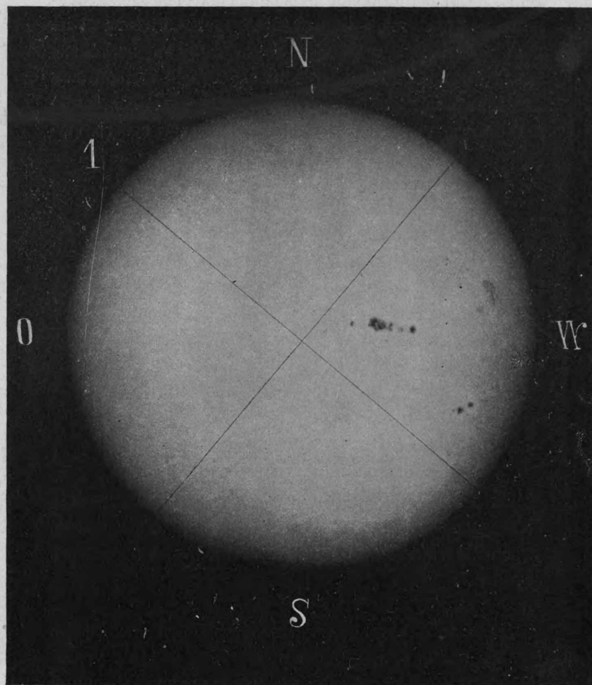
Иллюстрація 121. Солнечная пятна 14/27 іюня, 1905 г. въ 10 h 47 m 5. По фотографіи А. Ганскаго въ Пулковской обсерваторіи.
