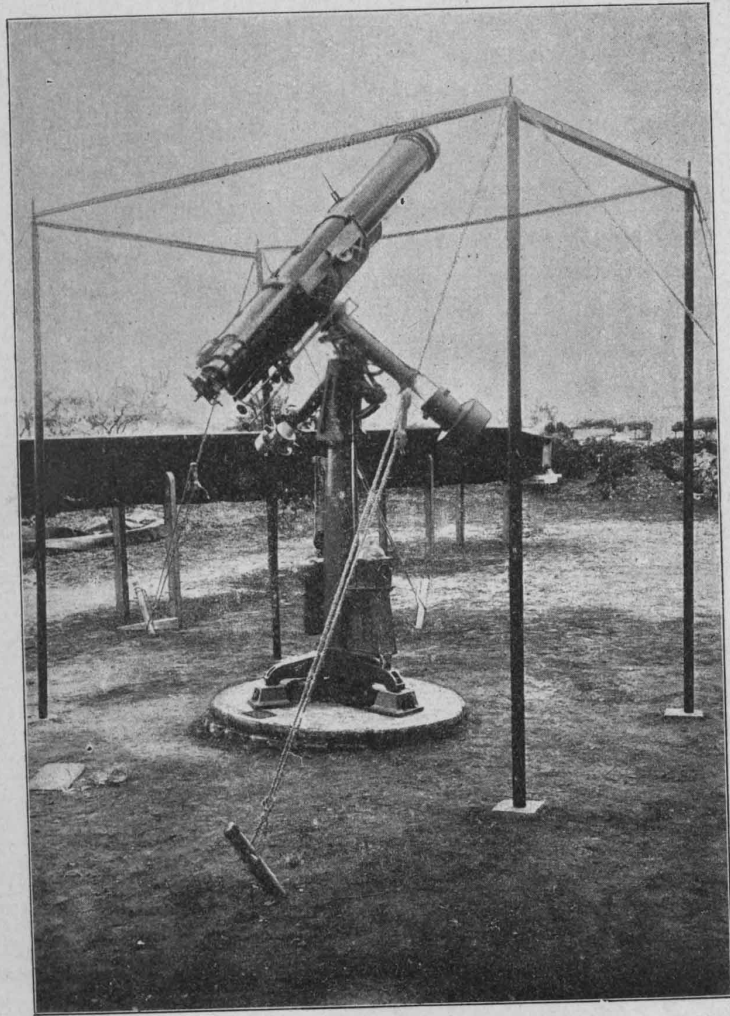
Иллюстрація 115. Въ ожиданіи солнечнаго затмѣнія. Приборъ для физическаго и химическаго изслѣдованія солнца.
