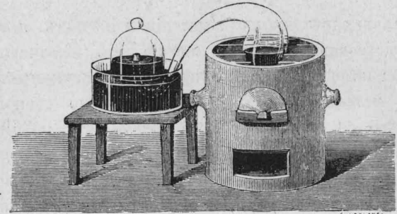
Иллюстрація 73. Аппарат Лавуазье для разложенія окиси ртути на металлъ и кислородъ (по рис. средины XIX вѣка).
