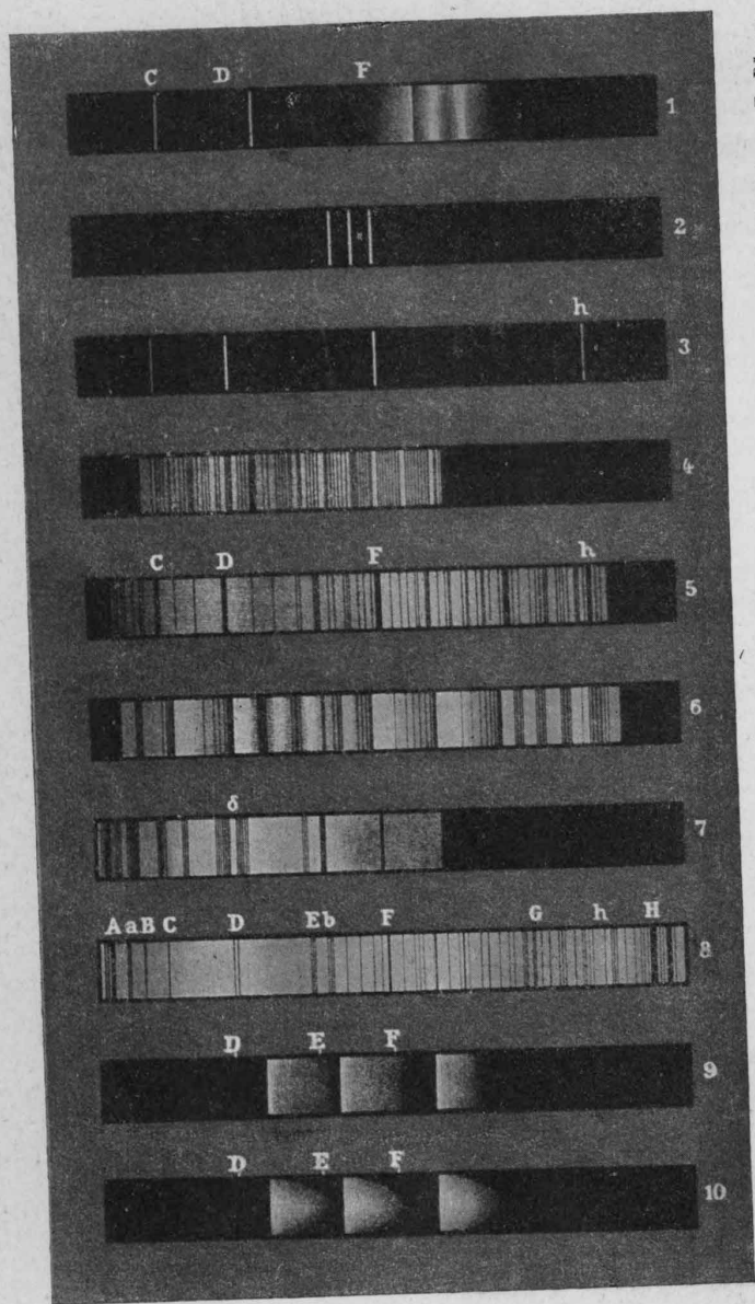
Иллюстрація . 113. Спектры. 1) Свѣрное сіаніе. 2) Туманности въ Драконѣ. 3) Протуберансы солнца. 4) звѣзды Т Вѣнга. 5) Спіріса (I типъ). 6) Альфа оріона (III типъ). 7) линии нашей атмосферы. 8) Спектръ солнца (II типъ). 9) Этилена. 10) Комета Виннеке 1868 г.
